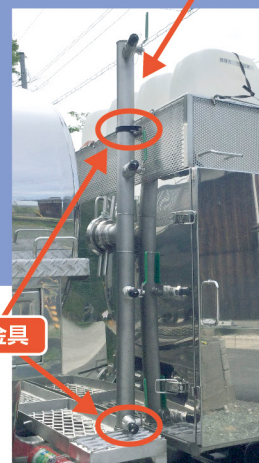
未使用時に給水タンク車に 固定した状態
